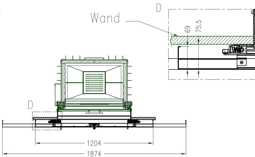
Horizontalschnitt M ~1:20
